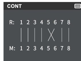
Pin5 & 6 cross
