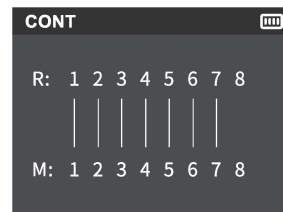
Pin8 Open
